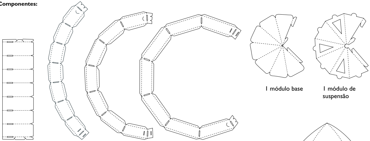
1 elemento base
