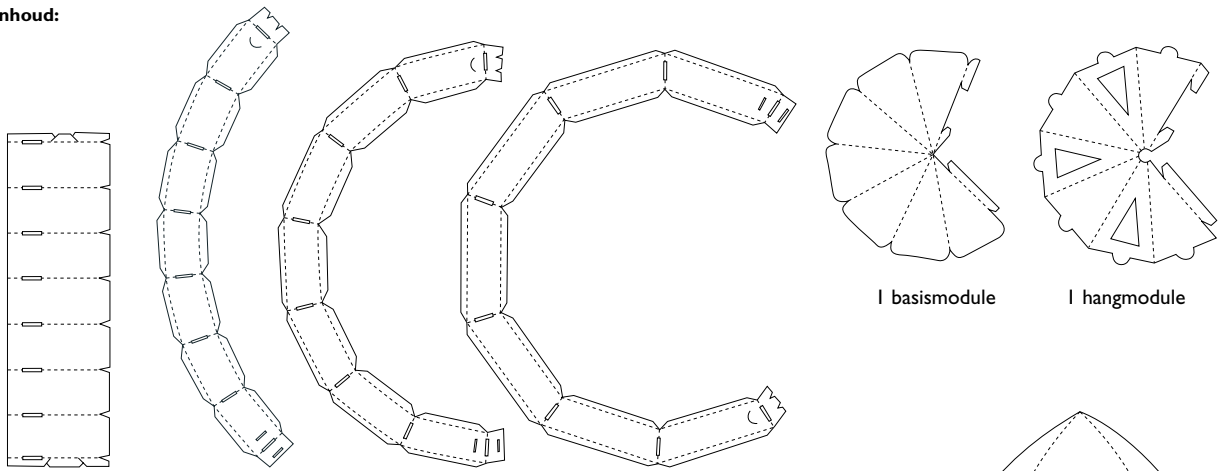
1 baselement
