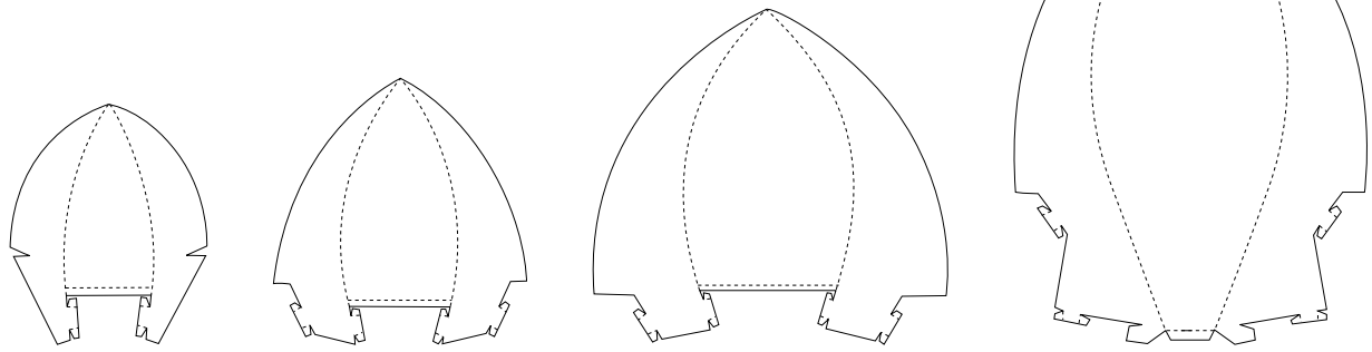
7 lampeskjermelementer, nr. 1
