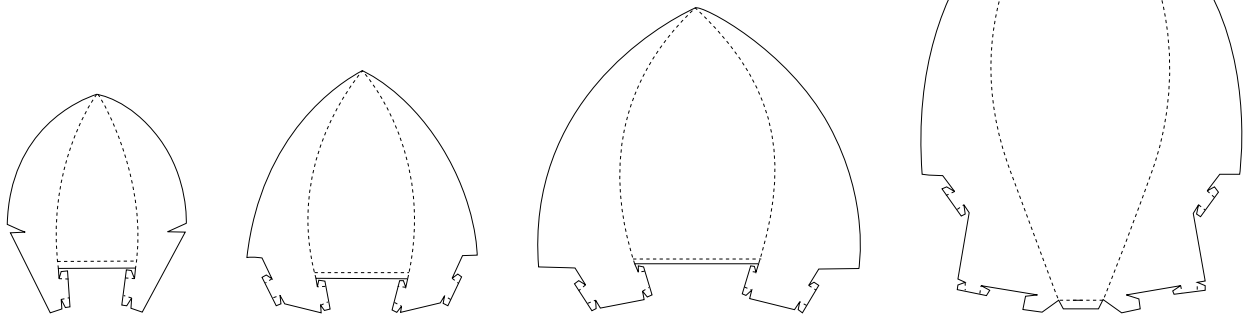
7 lampenkap-elementen nr. 1
