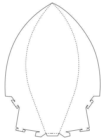
7 abats-jour n°4
